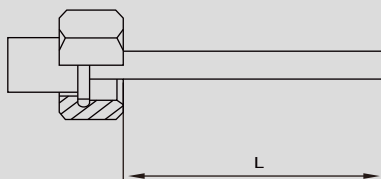
活動螺母牙
